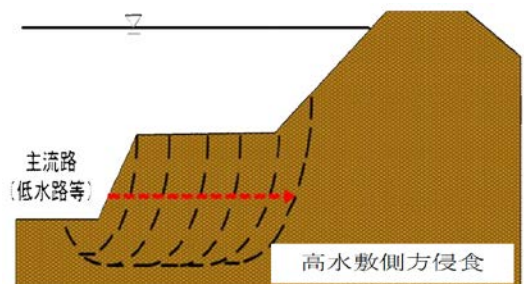
出水 (H23.9) で河岸侵食が進行し堤防が一部流出
